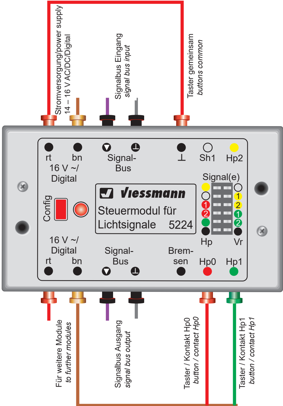
Beispiel einer Kabelbrückung Example of cable bridging
