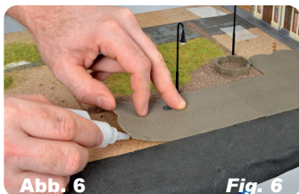
Abb. 6 Fig. 6 Untergrund mit Kleber einstreichen und Straßenplatte leicht andrücken.
