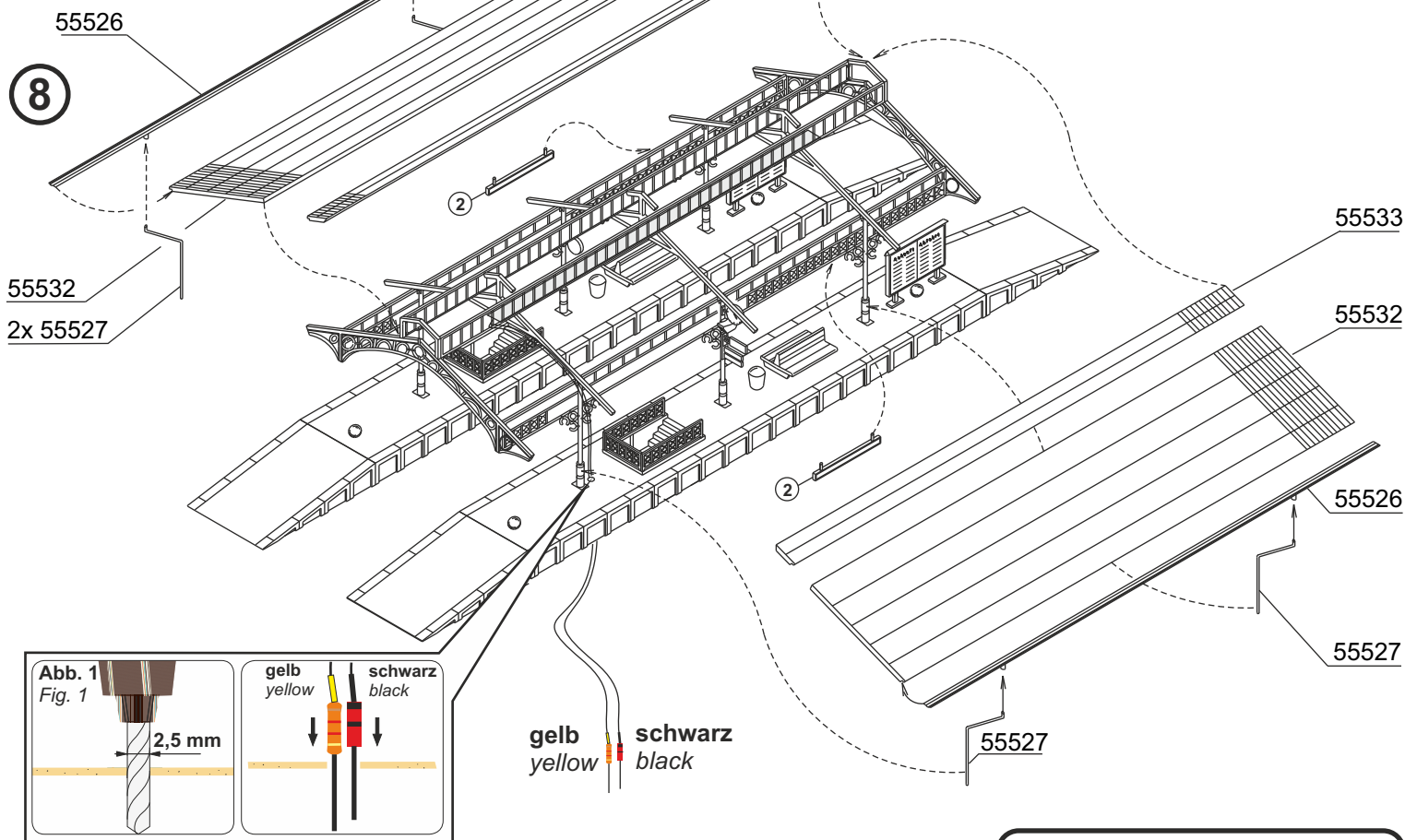
Abb. 1 Fig. 1 Am Einbauort ein Loch (Ø 2,5 mm) zur Montage bohren (Abb. 1). Drill a hole (Ø 2,5 mm) at the mounting place (fig. 1).
