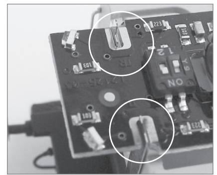
Löten / soldering / soudure / pájení / lutowanie
