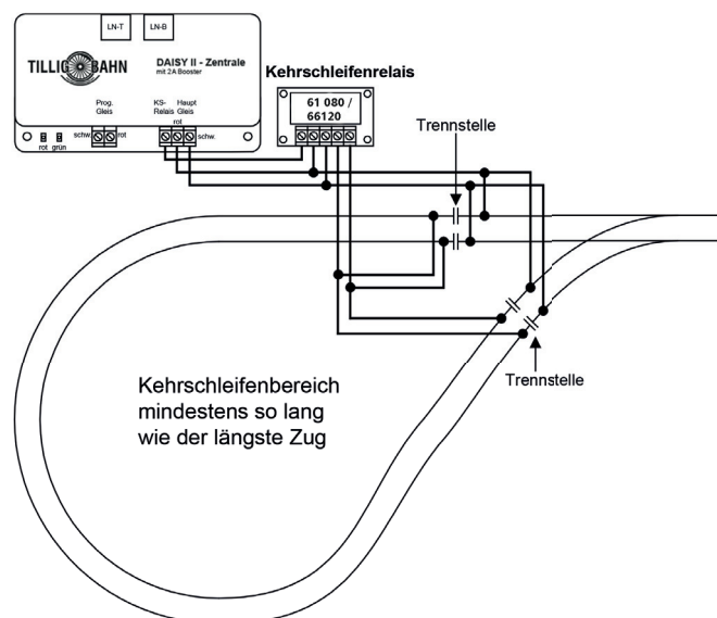
Anschlussplan eines Kehrschleifenrelais
