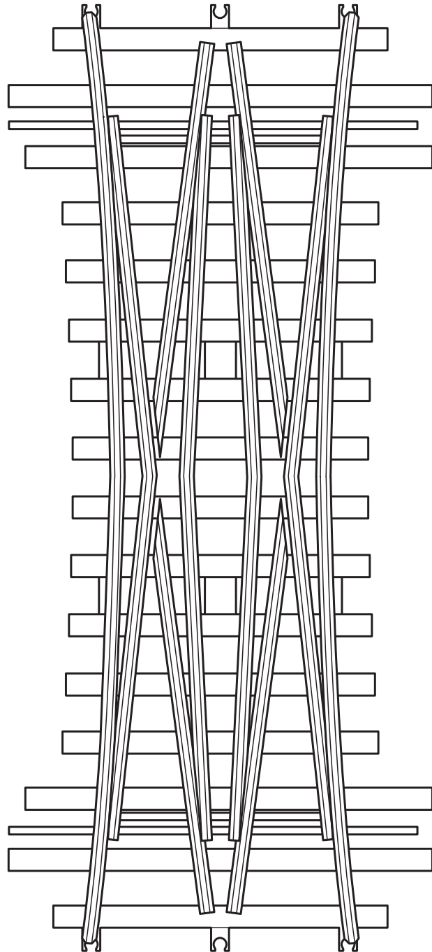
Doppelte Kreuzungsweiche - Mittelteil
